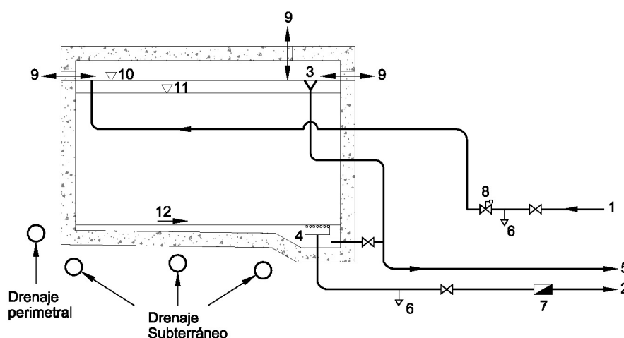
Esquema IV-1. Sección en alzado de un depósito
