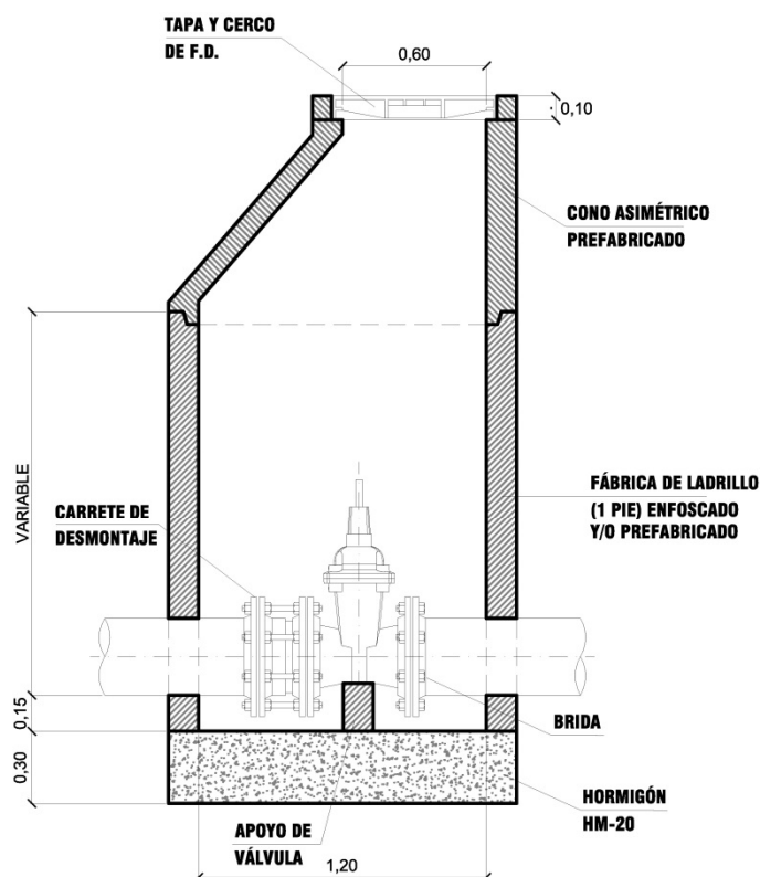
ALZADO SECCIÓN A-A
