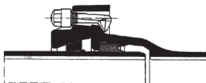
Unión acerojada
