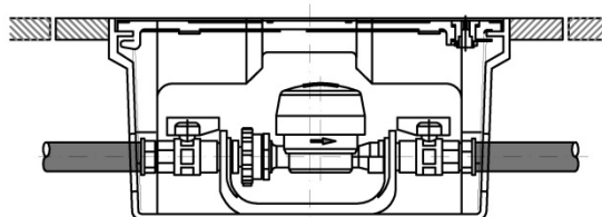
TRAMPILLÓN CON CONTADOR
