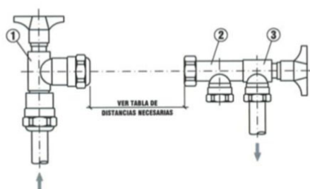
Esquema III-1. Alojamiento contador individual en armario
