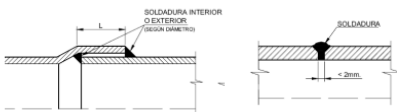
Unión abocardada
