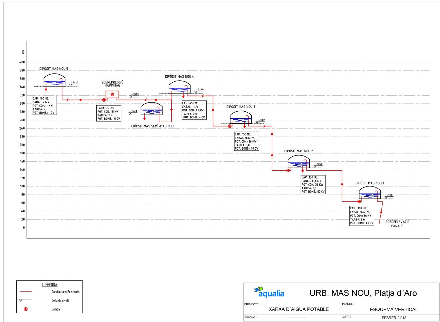
Il·lustració 3: Esquema vertical de la Urb. Mas nou de Platja d'Aro.
