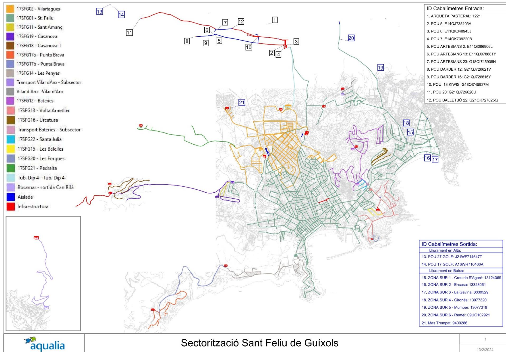
Il·lustració 1: Sectorització de la xarxa d'abastament de Sant feliu de Guíxols
