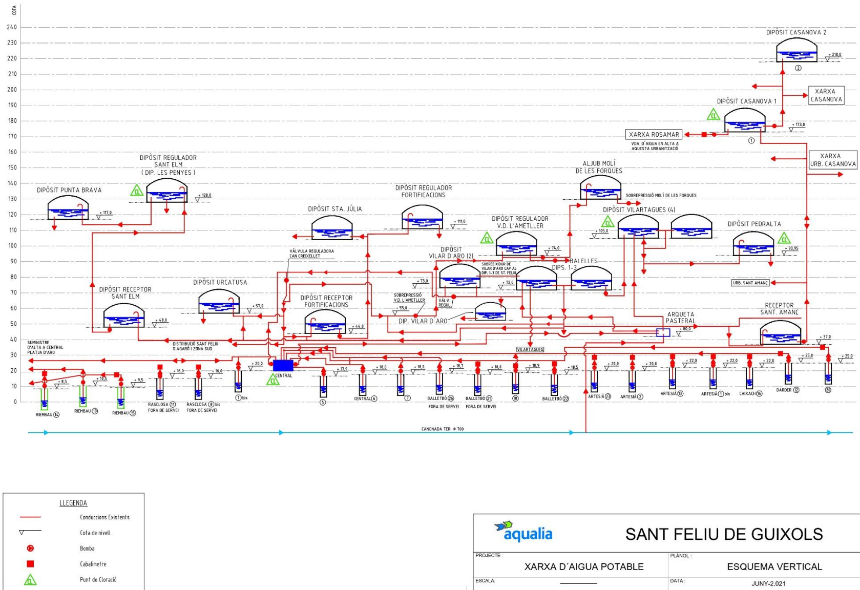
Il·lustració 2: Esquema vertical del servei de Sant Feliu de Guíxols
